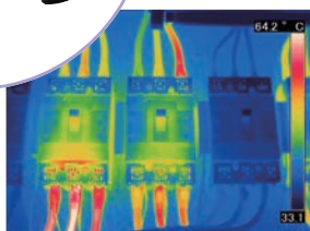
電気設備の発熱監視
