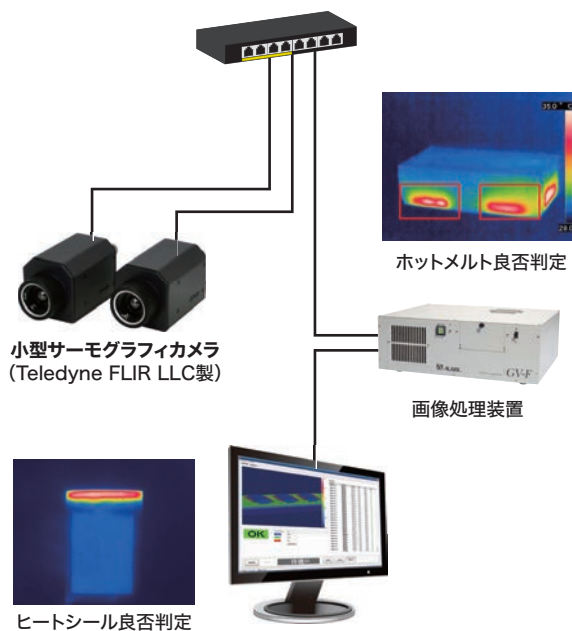
ヒートシール良否判定
