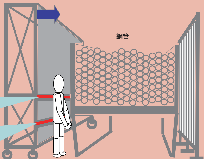
移動式玉掛け台
