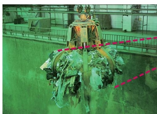
ごみピット
