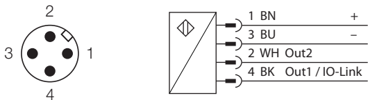
M12コネクタ ピンアサイン
