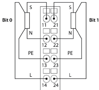
配線
