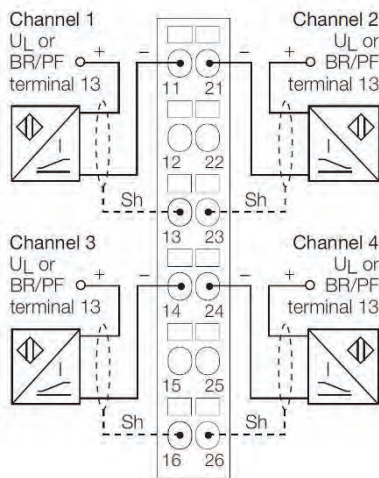
2線式センサ
