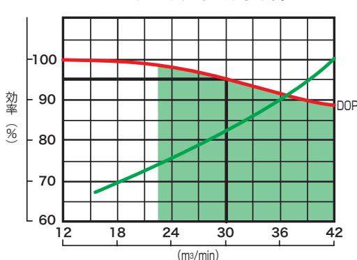
TRION T-Series 集塵効率(気流対効率) 30m 3 /min用セル
