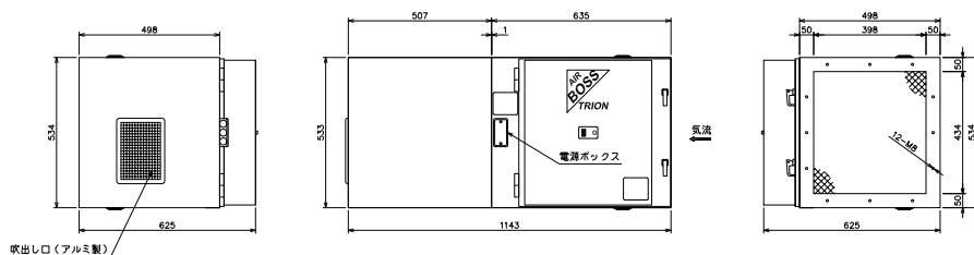
形 T1300-JYS 外形図 (参考)
